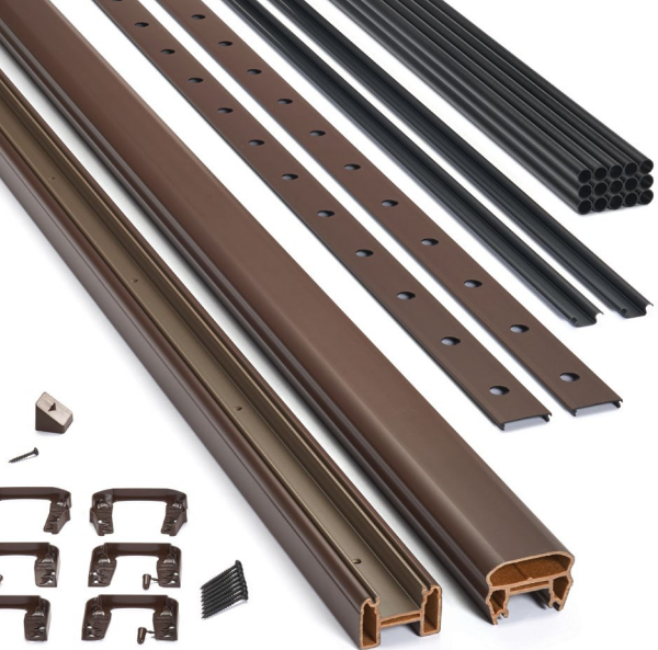
Nécessaire de rampe Transcend et balustres ronds en aluminium
