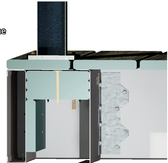
Side Rim Frame
